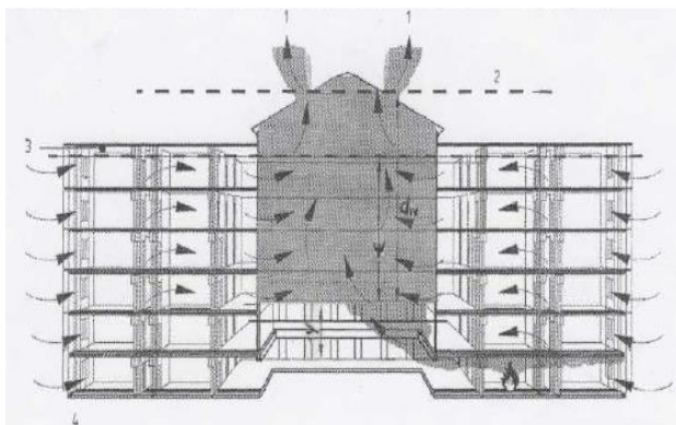
Figura 2. Principiul sistemului de ventilație care protejează căile de evacuare (PNP deasupra celui mai de sus etaj). 1 – deschidere de ventilație; 2 – linia centrală a deschiderilor de ventilație ( C_v A_v ); 3 – plan neutru de presiune; 4 – admisia ( C_i A_i ).
