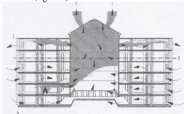
Figura 1. Plan neutru de presiune – ventilare longitudinală. 1- deschidere de ventilare; 2 – scurgere; 3 – plan neutru de presiune; 4 – orificiu de admisie egal cu orificiu de evacuare
