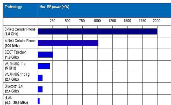
Fig.3 Puterea de emisie la diferite benzi de frecvență
