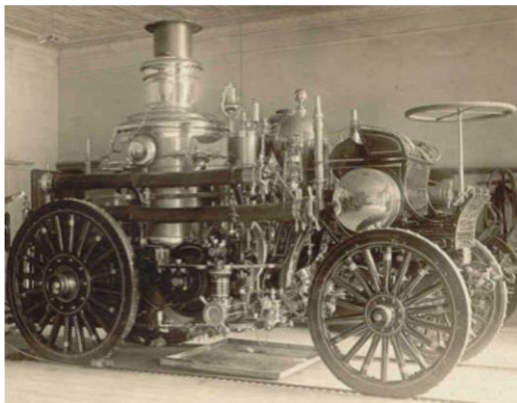
Fig. 1. Vehicul acționat de motor cu abur.
