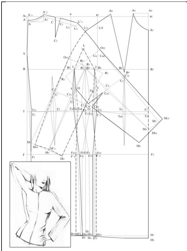
Figura 4. Produs de croială chimono cu clinul lateral al produsului croit separat și pavă
