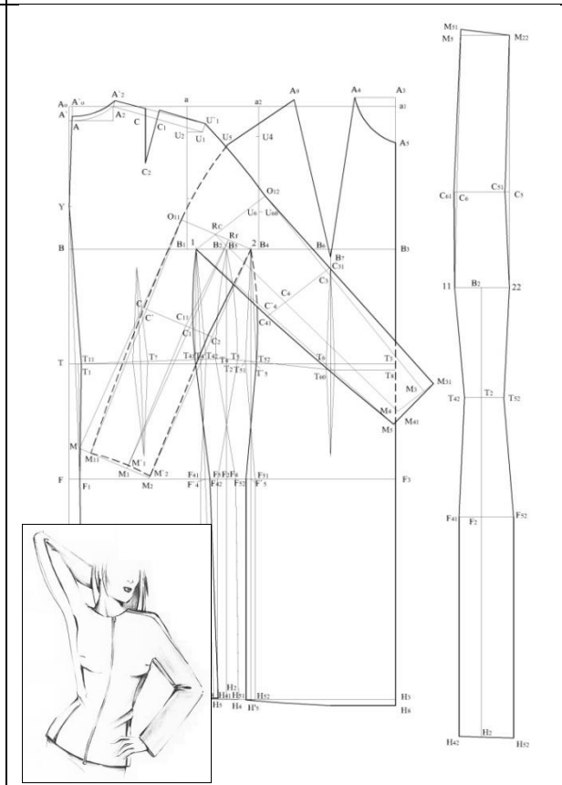
Figura7. Produs de croială chimonocu clin și partea inferioară a mânecii indivizibilă
