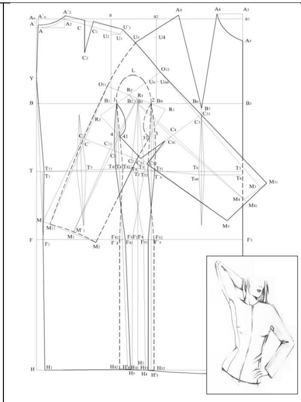
Figura5. Produs de croială chimono cu clunul lateral al produsului croit separat și pavă de formă ovală
