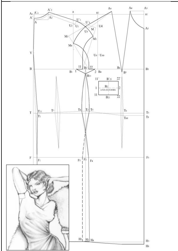
Figura6. Produs de croială chimono scurtă cu pavă dreptunghiulară
