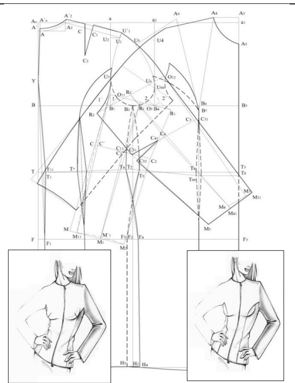
Figura 9. Produs de croială chimono cu prelungire în răscoiala mânecii clasice și linie de „relief”
