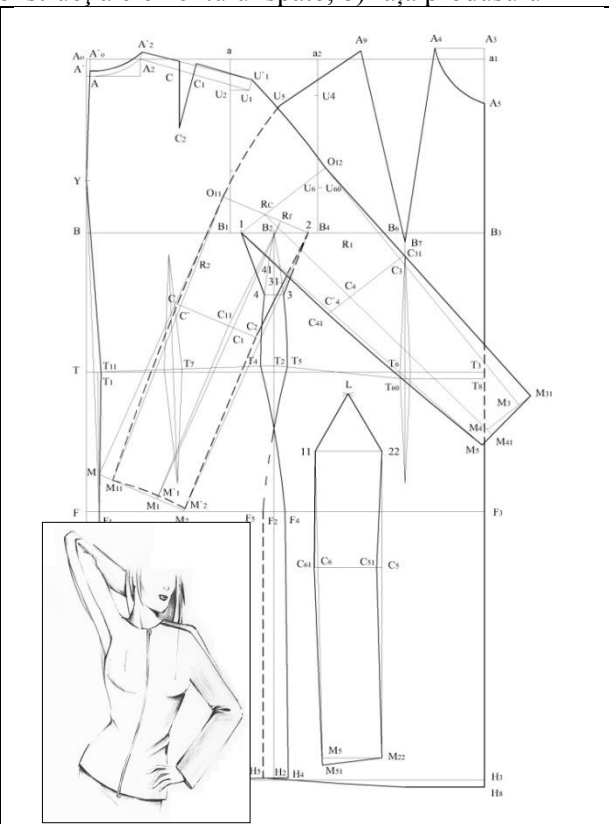
Figura 3. Produs de croială chimono cu partea inferioară a mânecii croită separat și pavă
