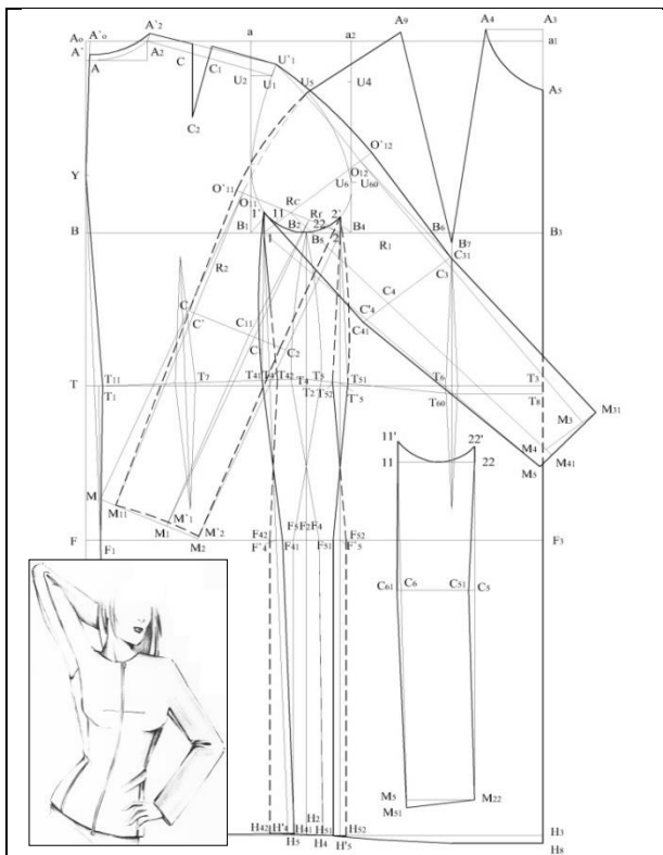
Figura 8. Produs de croială chimono cu prelungire în răscoiala mânecii clasice cu clinul lateral al produsului și partea inferioară a mânecii croite separat
