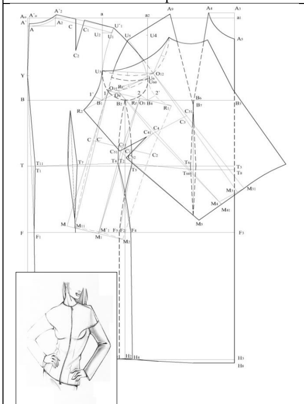
Figura 10. Produs de croială chimono cu prelungire în răscoiala mânecii clasice cu un sector al mânecii croit separat
