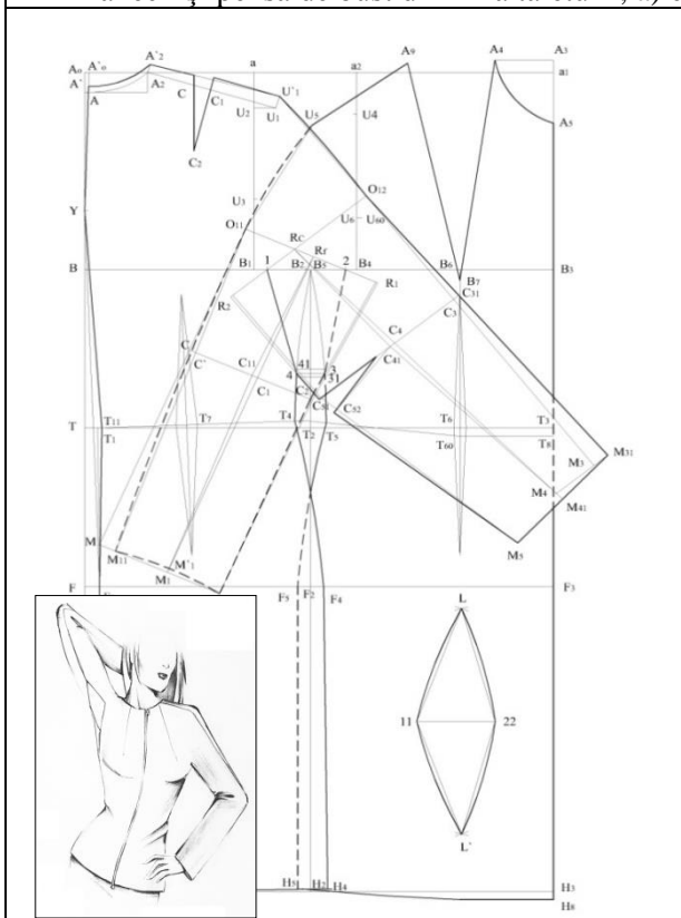
Figura 2. Produs de croială chimono cu pavă în formă de romb
