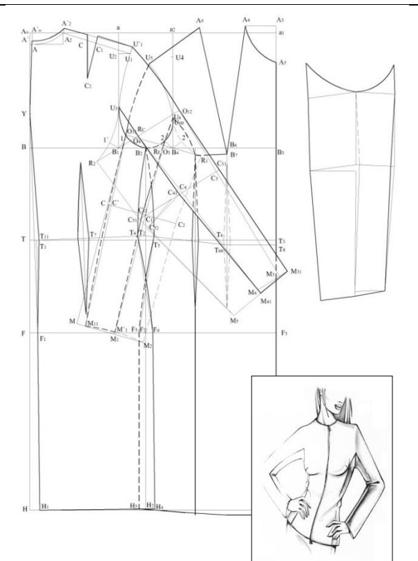
Figura 11. Produs de croială chimono cu prelungire în răscoiala mânecii clasice și partea inferioară a mânecii croită separat
