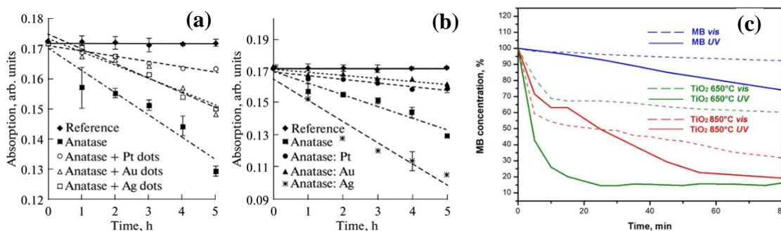
Fig. 5. Dependența absorbției în timp în urma excitării cu lumina UV pentru probele de TiO 2 cu faza anatase: (a) dopate cu Au, Ag sau Pt, (b) funcționalizate cu nanodote metalice și (c) procesul de degradare a compusului MB în timp sub iradierea cu lumina UV sau vizibilă [4,11].
