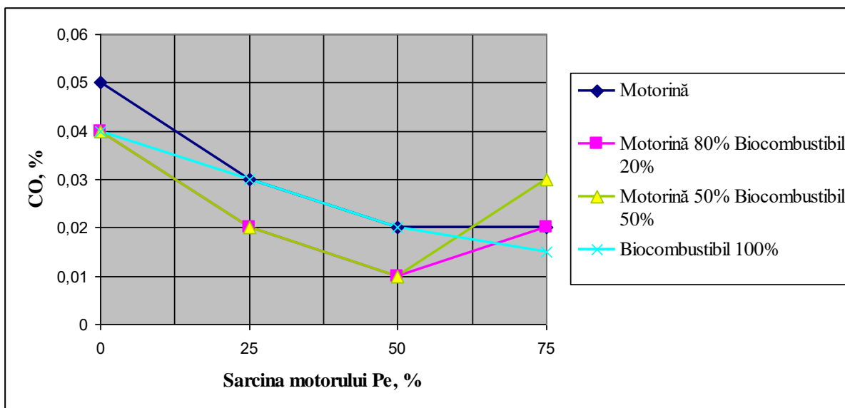
Fig. 1. Emisia de CO în gazele de eșapament în dependență de sarcina motorului.
