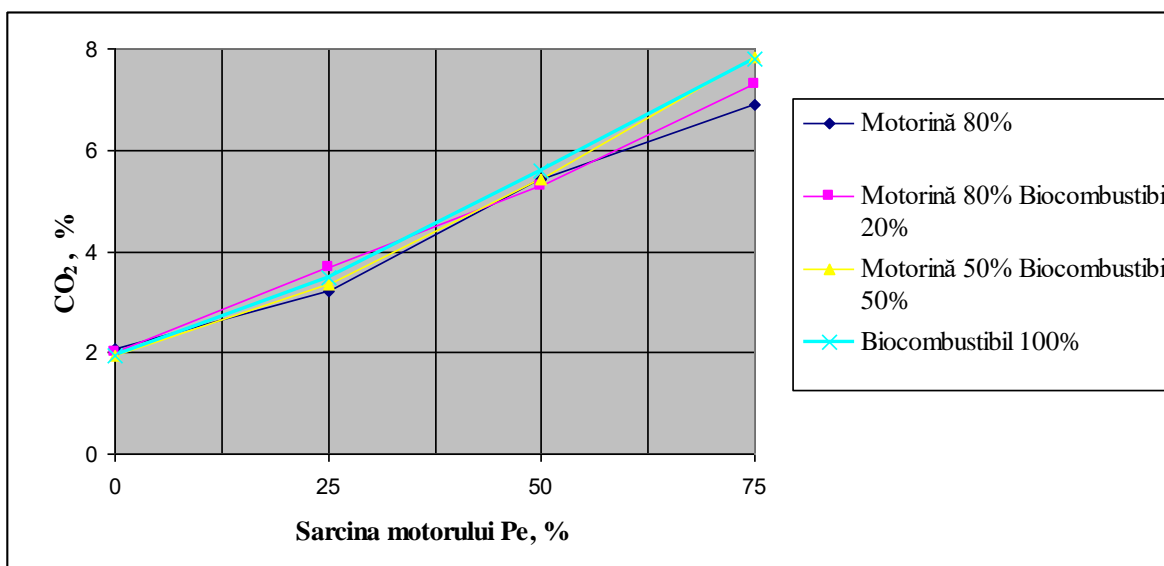
Fig. 2. Emisia de CO 2 în gazele de eșapament în dependență de sarcina motorului.
