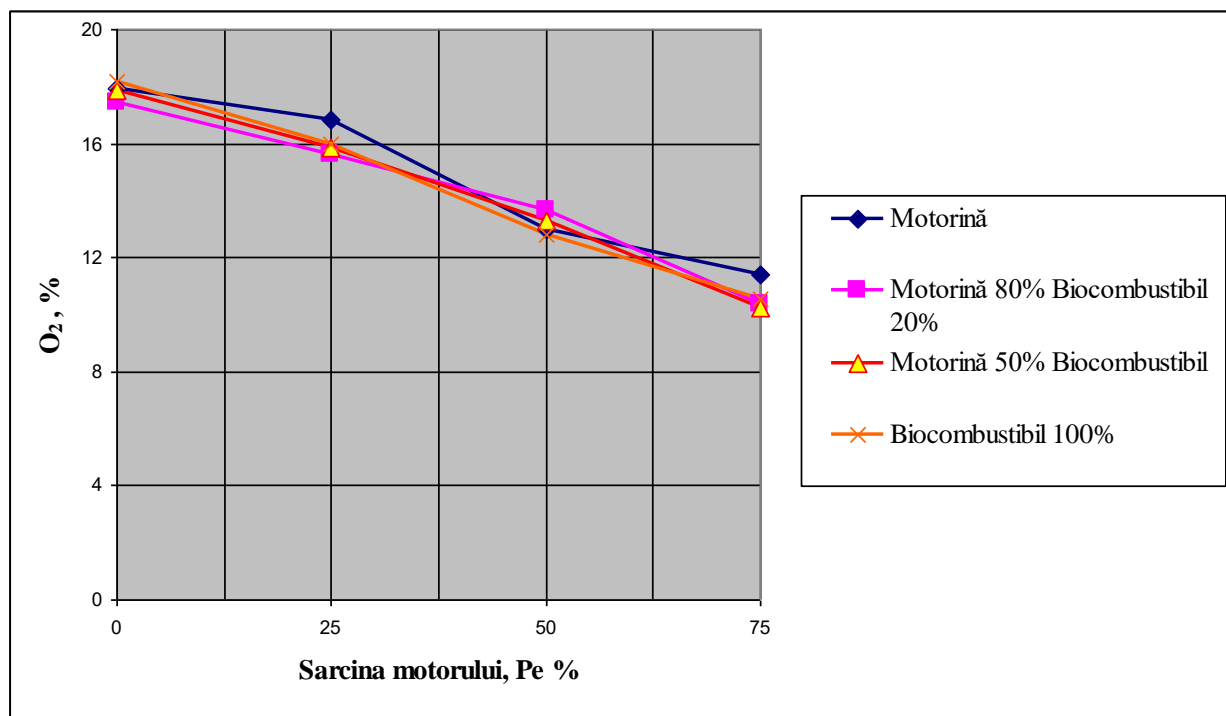
Fig. 4. Emisia de O 2 în gazele de eșapament în dependență de sarcina motorului.
