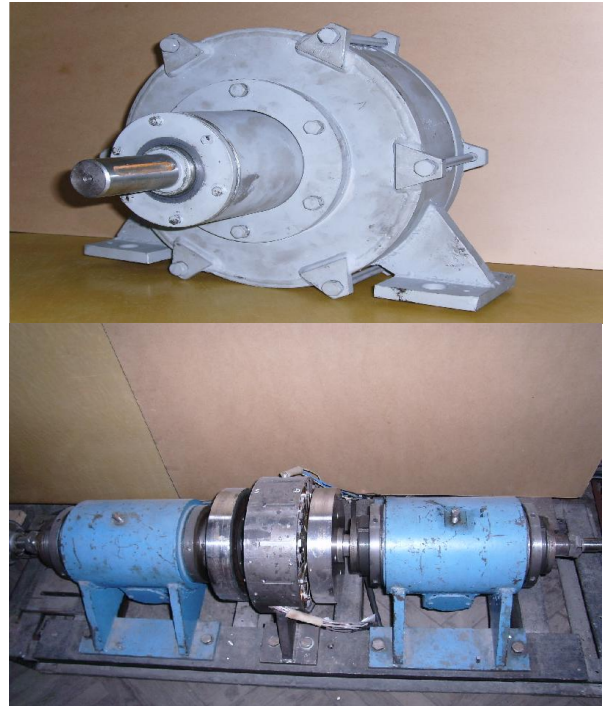
Fig 12 Modele de generatoare cu flux magnetic axial elaborate în cadrul catedrei
